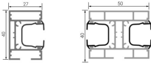
Einzelführungsschiene Doppelführungsschiene
